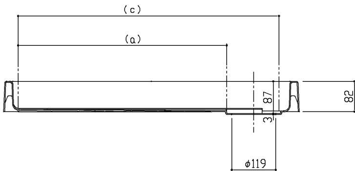
断面A-A
